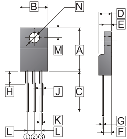
ITO-220
