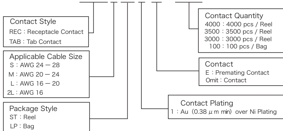
Tab Contact
