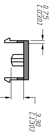
DETAIL A-A
