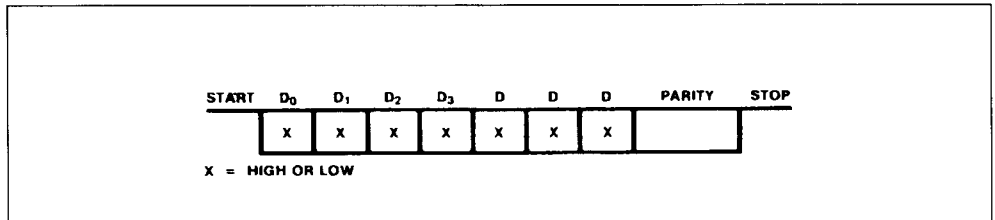
Figure 7 : Asynchronous Message Format.
