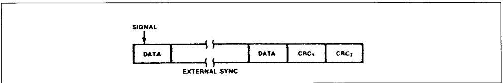
Figure 11 : SDLC Message Format.
