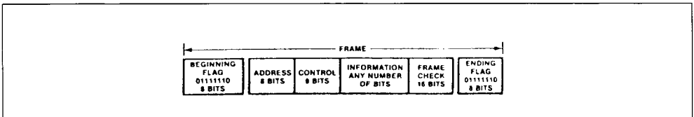
Figure 11 : SDLC Message Format.
