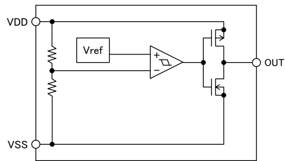
CMOS Output
