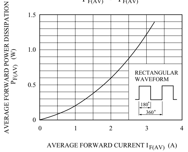
P_{F(AV)} - I_{F(AV)}
