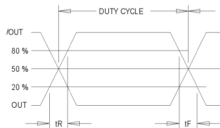
Output Waveform: LVDS / CML / LVPECL
