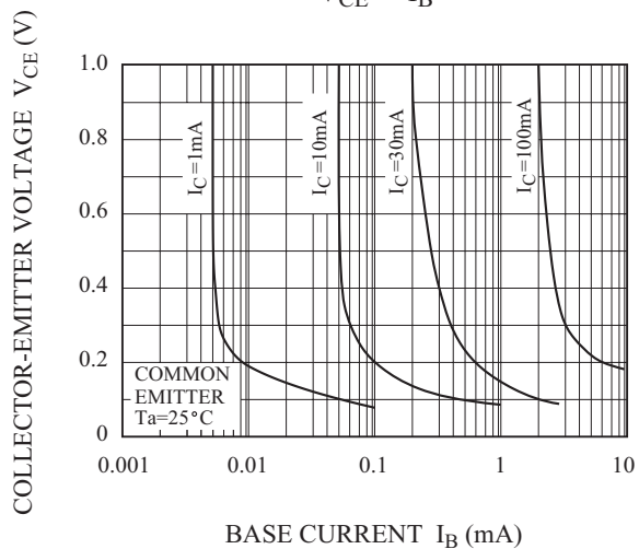
V_{CE} - I_B
