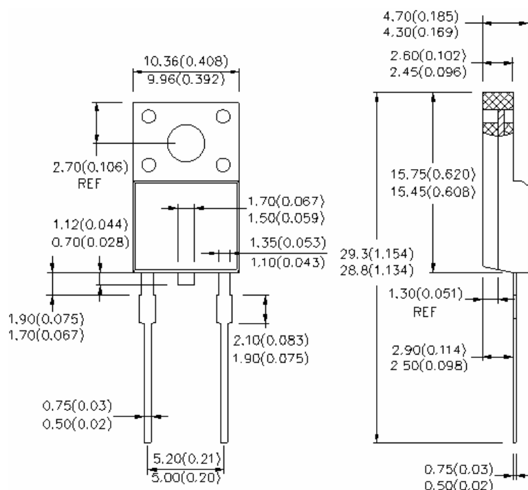
ITO-220AC
