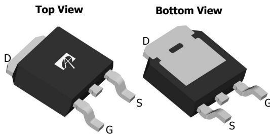
TO252 DPAK
