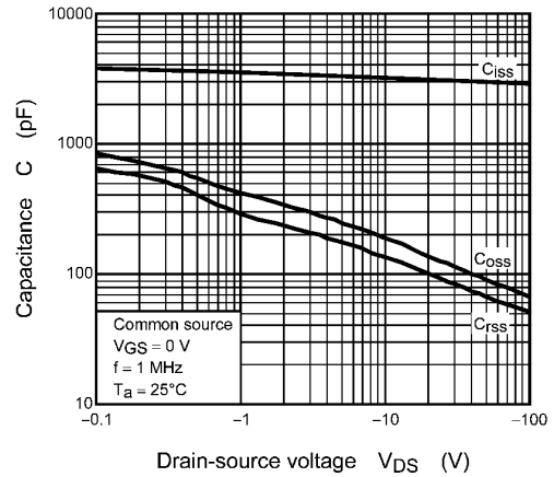
Fig. 8.8 Capacitance - V_{DS}
