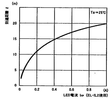
■到達距離/LED電流特性 \ell/I_{FP}
