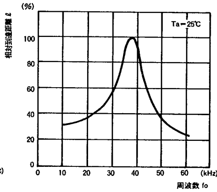
■到達距離/周波数特性 \ell/f_o
