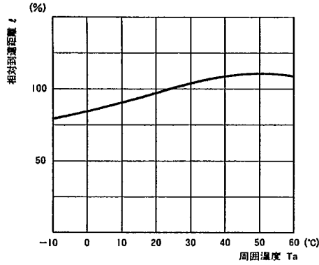
■到達距離/周囲温度特性 \ell/T_a
