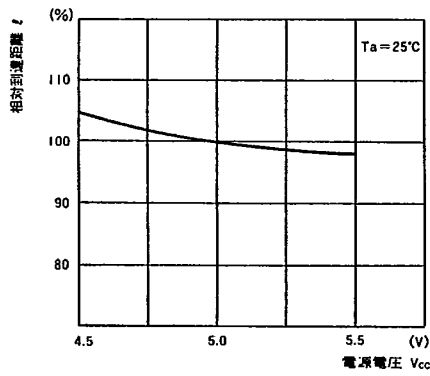
■到達距離/電源電圧特性 \ell/V_{CC}
