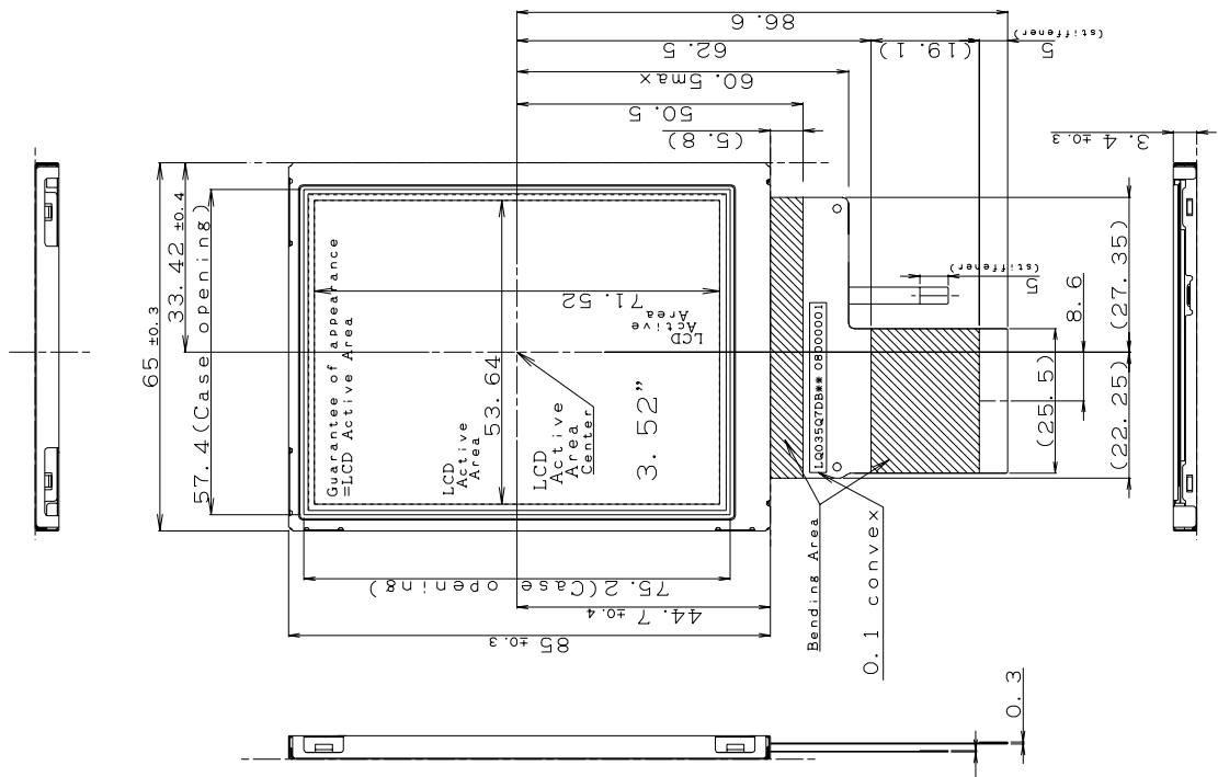
図 1 外形寸法図
