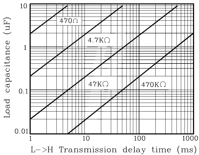
Fig. 9 C_L - t_{PLH}
