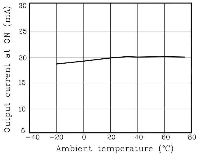
Fig. 7 I_{OL} - T_a
