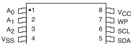
TSSOP Package (U)
