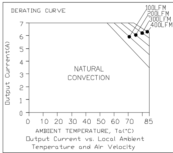
Vin=48 V, Vo=12 V
