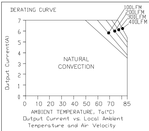
Vin=24 V, Vo=12 V
