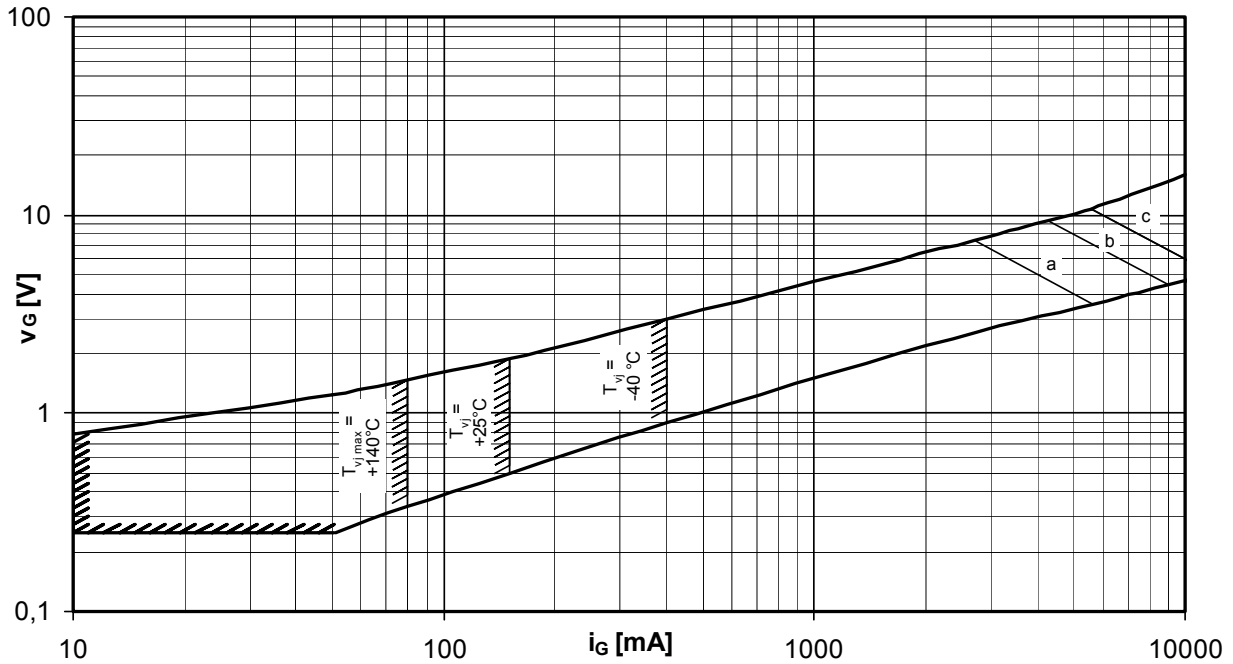
Steuercharakteristik v_G = f(i_G) mit Zündbereichen für V_D = 12\text{ V} Gate characteristic v_G = f(i_G) with triggering area for V_D = 12\text{ V}
