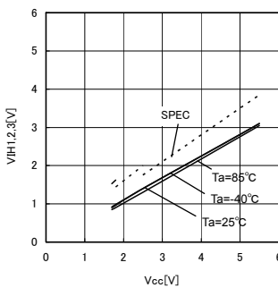
Fig.4 H input voltage VIH1,2,3 (A2,SCL,SDA,WP)
