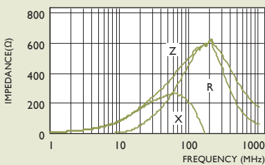
PBY160808T-501Y-S
