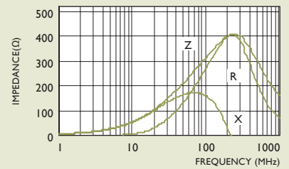
PBY160808T-301Y-S
