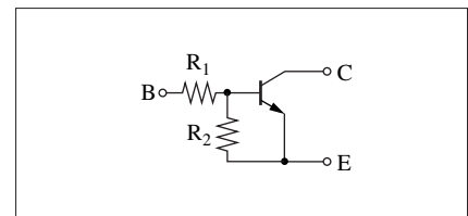
内部接続図
