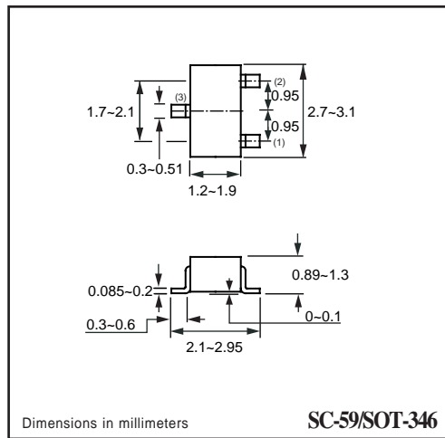
SC-59/SOT-346
