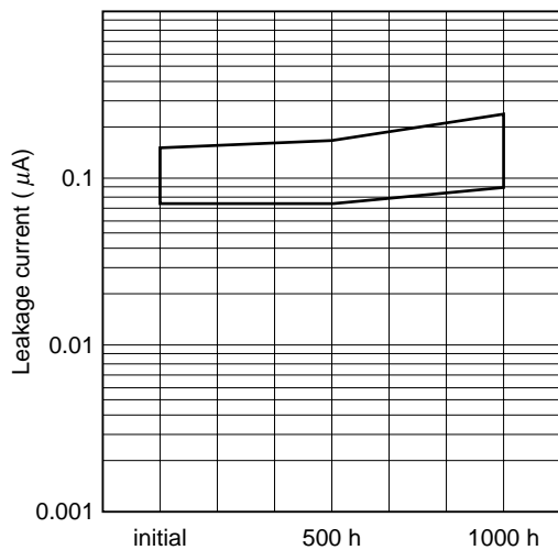
10 V/33 μF
