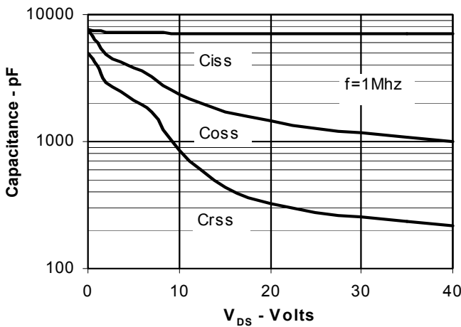
Fig. 11. Capacitance
