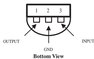
TO-92 (N)
