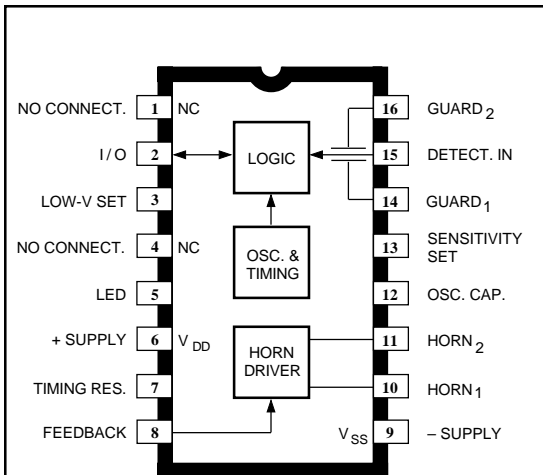
Dwg. PC-004-1
