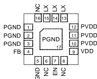
WQFN-16L 3x3
