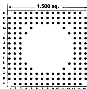
149 PINS Footprint 15019
