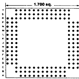
145 PINS Footprint 17004
