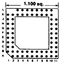
Footprint 11034
