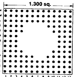
133 PINS Footprint 13048
