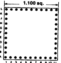
Footprint 11044
