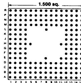
181 PINS Footprint 15033
