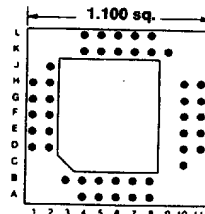
Footprint 11041
