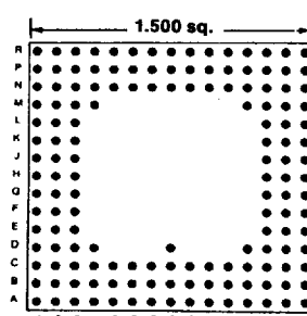
149 PINS Footprint 15035
