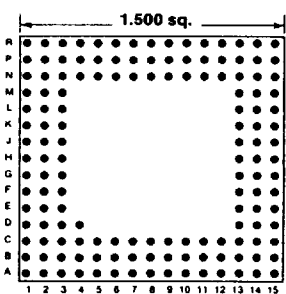
145 PINS Footprint 15024
