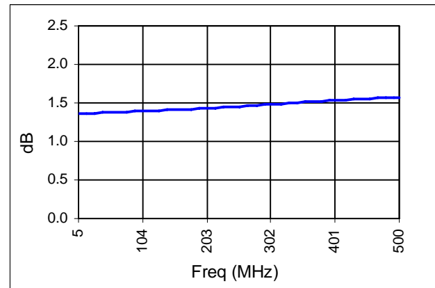
IF VSWR
