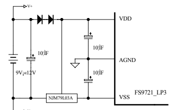
图 13 9V~12V 电源供电
