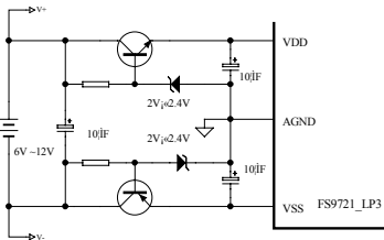
图 12 6V~12V 电源供电
