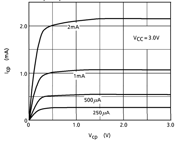
V cp - I cp CHARACTERISTICS PLL2 Nch
