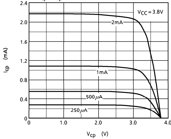
V cp - I cp CHARACTERISTICS PLL1 Pch
