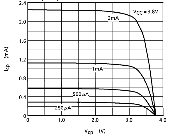
V cp - I cp CHARACTERISTICS PLL2 Pch
