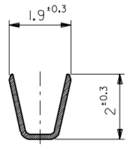
SECT.D-D
