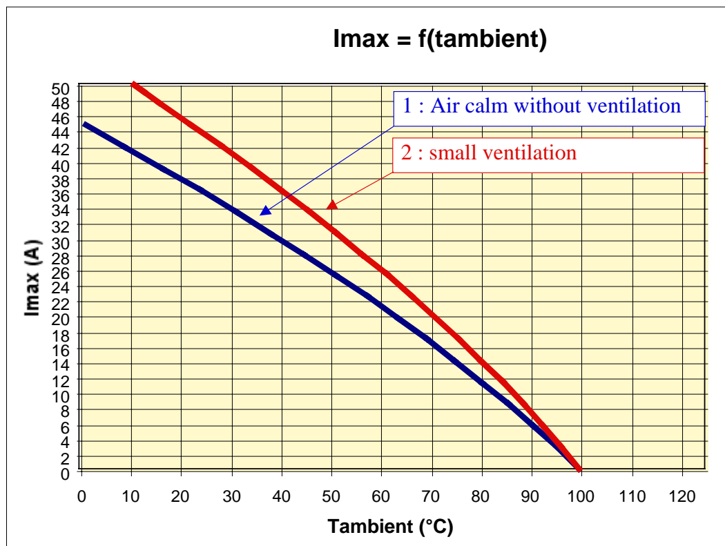
Fig. 2 Courbes thermiques & Choix dissipateur thermique / Thermal curves and heatsink choice
