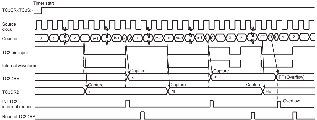
a) TC3SEL<TC3INV>=0
