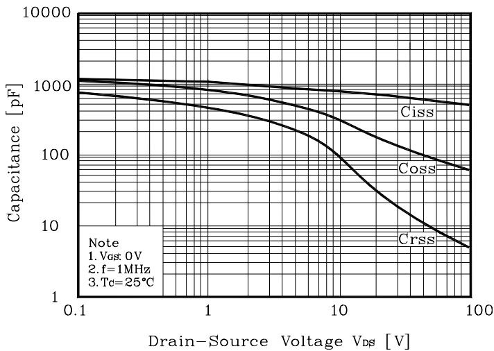
Fig. 5 Capacitance - V_{DS}
