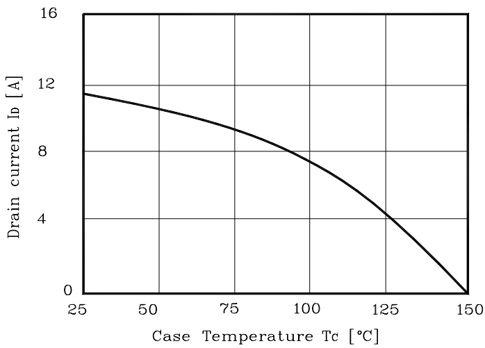
Fig. 9 I_D - T_C
