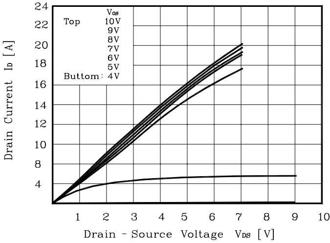
Fig. 1 I_D - V_{DS}
