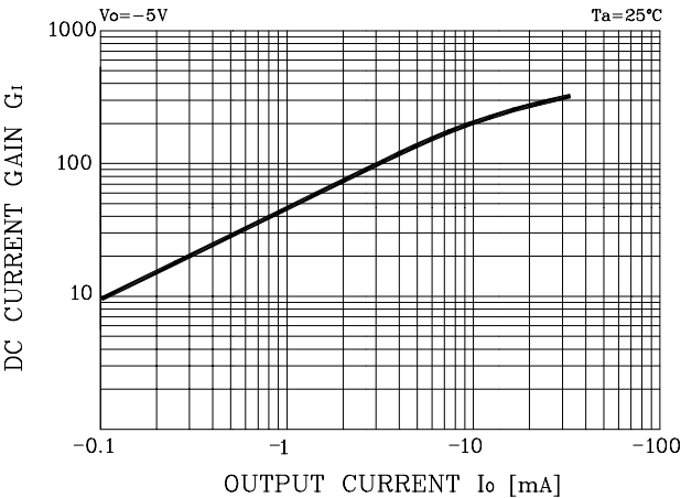
Fig. 3 G_1 - I_o
