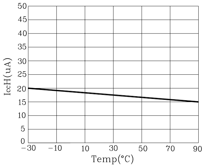
Fig. 3 I_{CCH} - Temp
