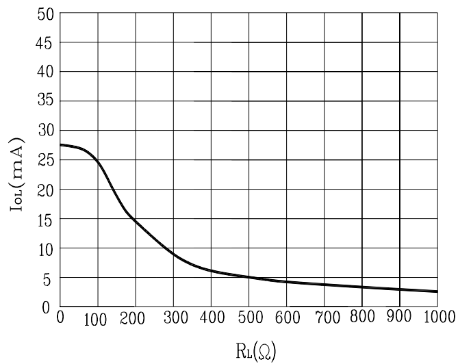
Fig. 4 I_{OL} - R_L
