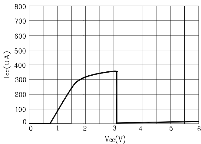
Fig. 2 I_{CC} - V_{CC}
