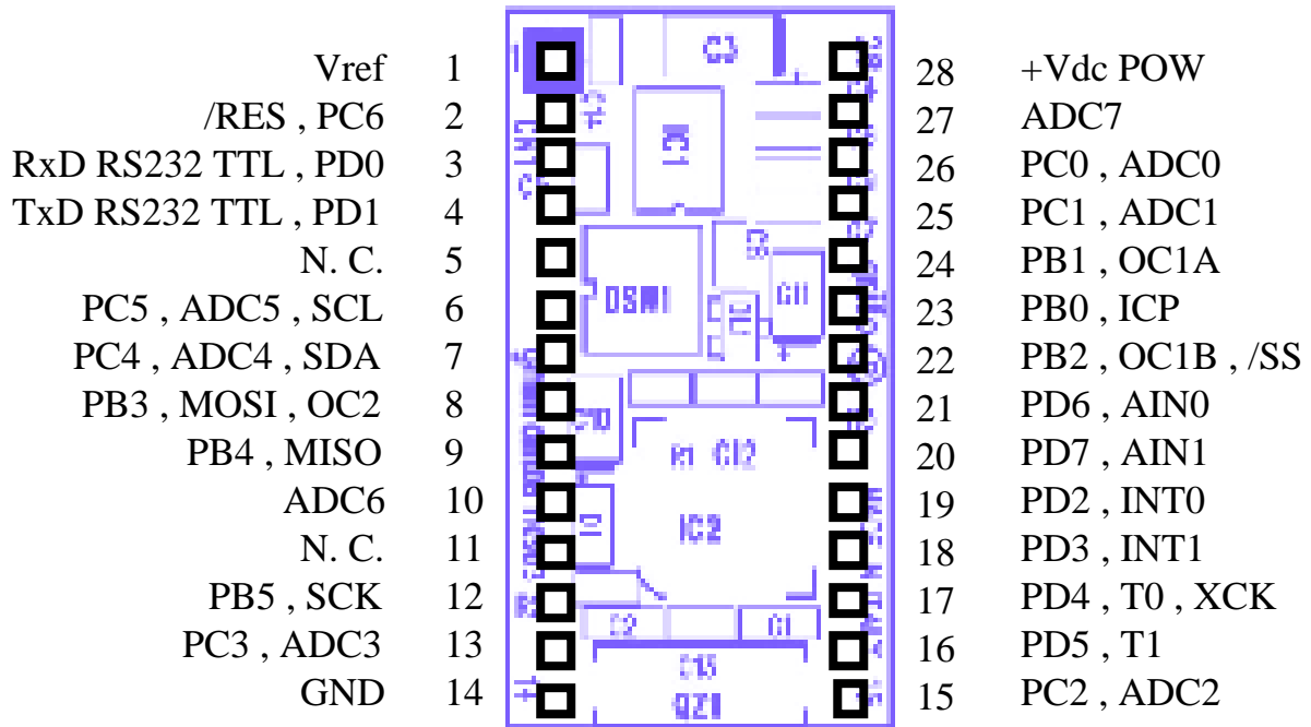
FIGURA 5: CN1 - ZOCCOLO CON SEGNALI DEL MINI MODULO
