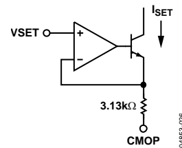
Figure 27. VSET Interface
