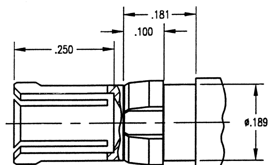
Receptacle Interface
