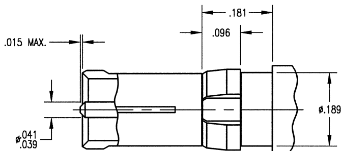
Receptacle Interface
