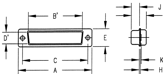
Receptacle Shell
