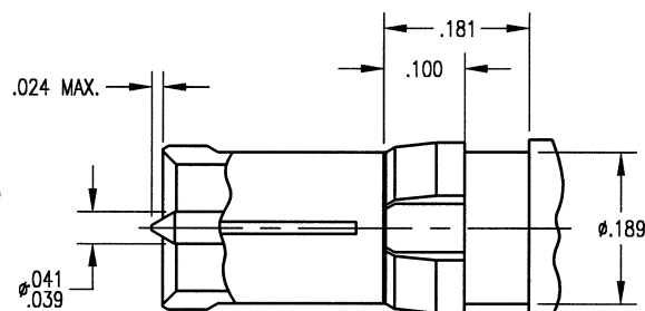
Receptacle Interface
