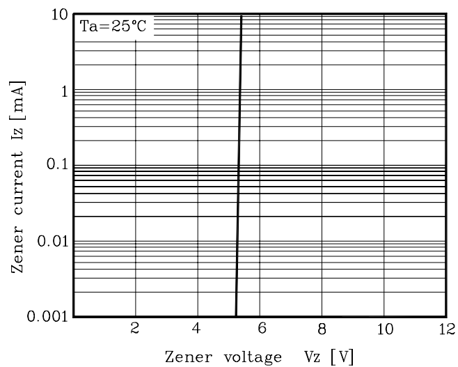
Fig. 2 I_Z - V_Z
