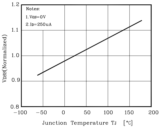
Fig. 7 V_{DSS} - T_J
