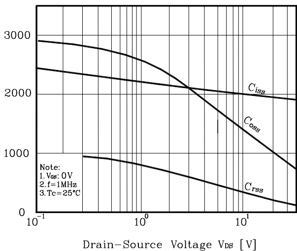
Fig. 5 Capacitance - V_{DS}
