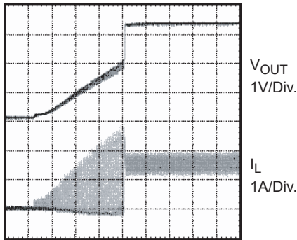
4ms/Div. VIN = 12V, VOUT = 3.3V, RLOAD = 2Ω
