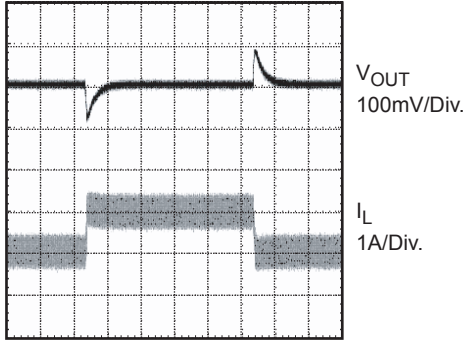
200µs/Div. VIN = 12V, VOUT = 3.3V, 1A - 2A STEP
