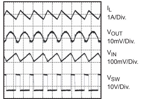
2µs/Div. VIN = 12V, VOUT = 3.3V, RLOAD = 2Ω
