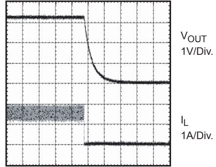
100µs/Div. VIN = 12V, VOUT = 3.3V, RLOAD = 2Ω
