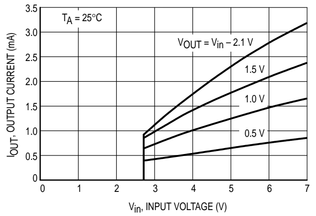
MC33461-4.5
