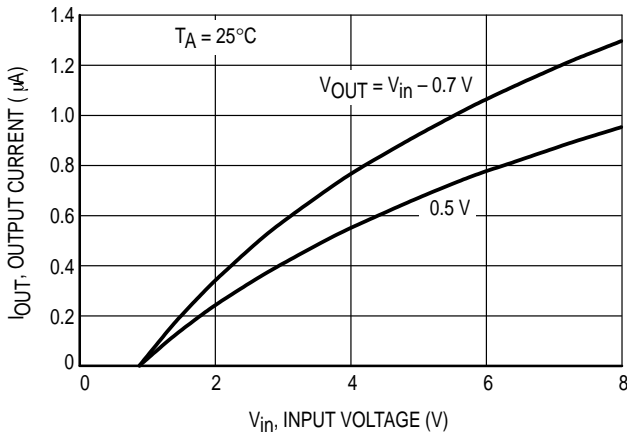
MC33461-0.9
