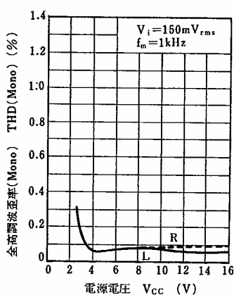
THD(Mono) - V_{CC}
