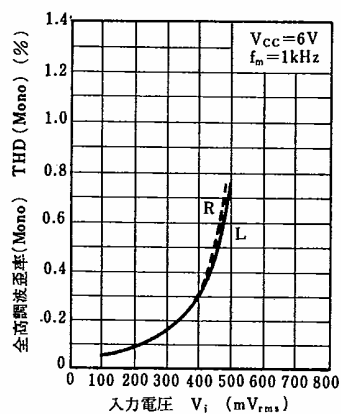
THD(Mono) - V_i
