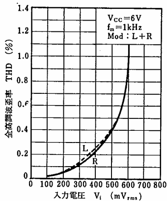
THD - V_i
