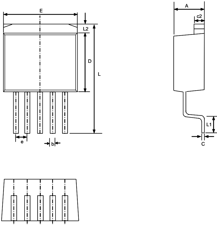
TO-263-5 Package
