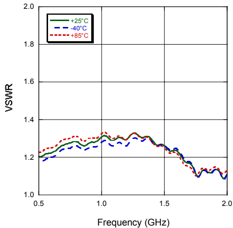
VSWR
