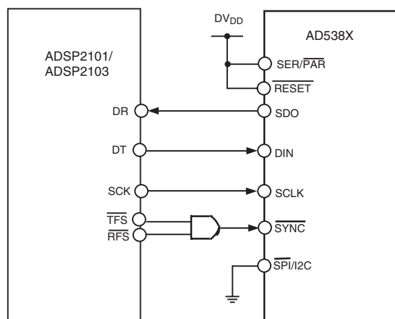
Figure 18. AD5380 -ADSP2101/ADSP2103 Interface
