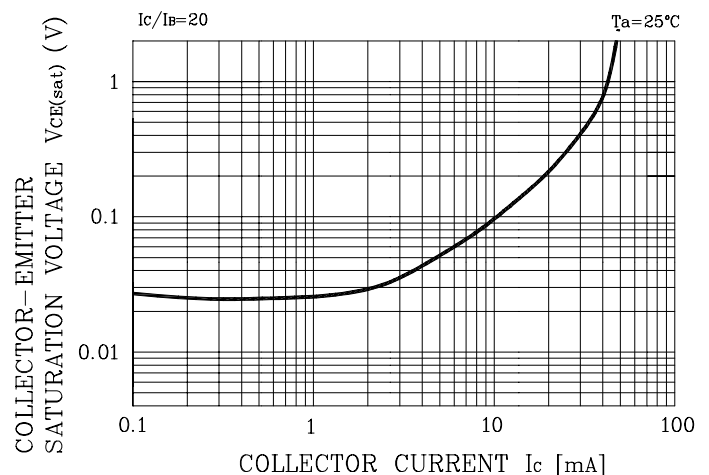
Fig. 2 V_{CE(SAT)} - I_C
