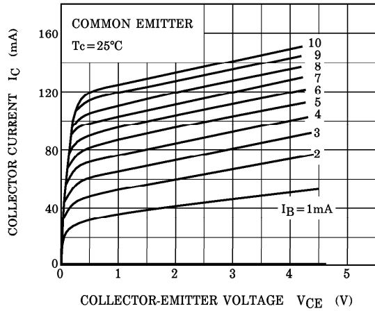
I_C - V_{CE}
