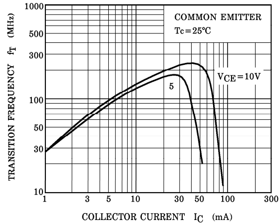
f_T - I_C
