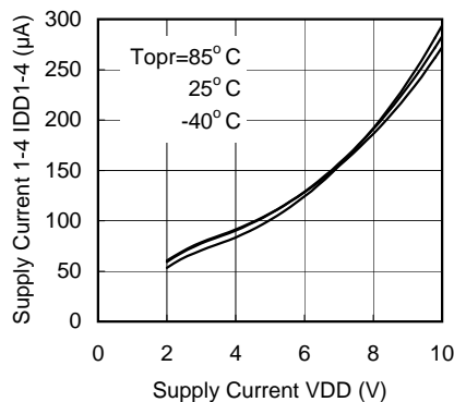
XC9505B092 (180KHz)
