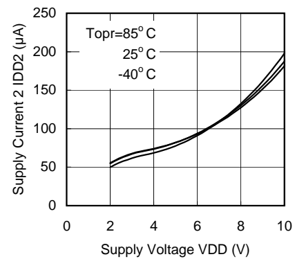
XC9505B092 (180KHz)
